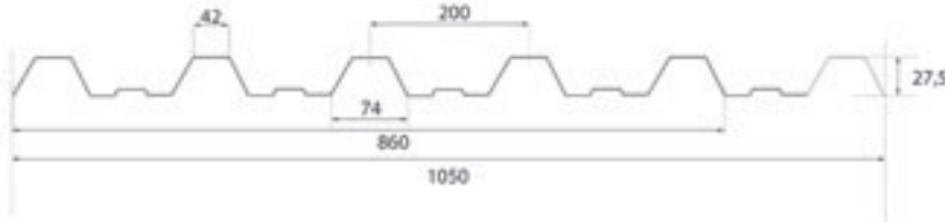
Trapezli Galvanizli Sacların Taşıyabileceği Yayılı Yükler (KG/M2)
